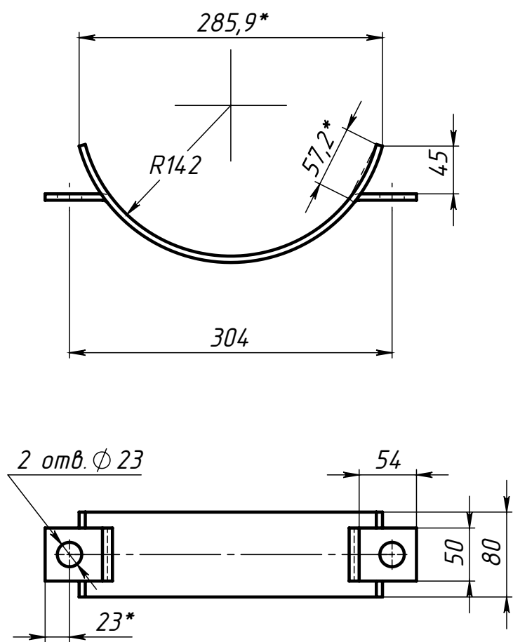
Поз.3 (Подушка)
