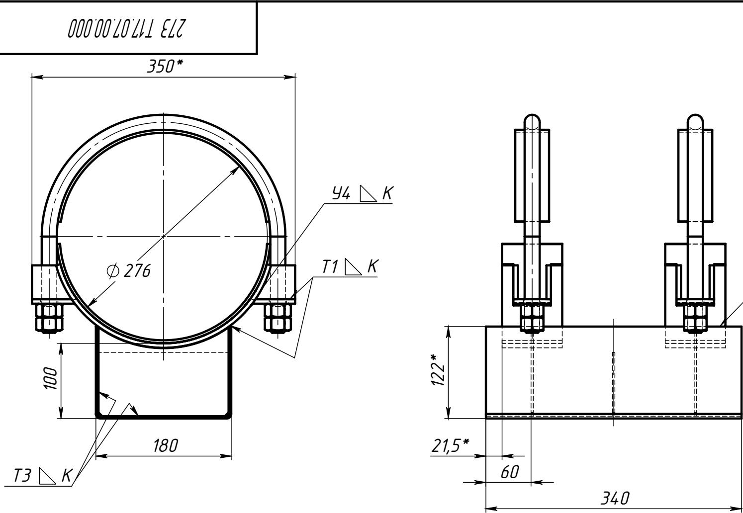
Поз.3 (Подушка)
